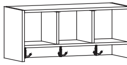
36w x 14d x 16h #WCB2584 Wgt- 43
